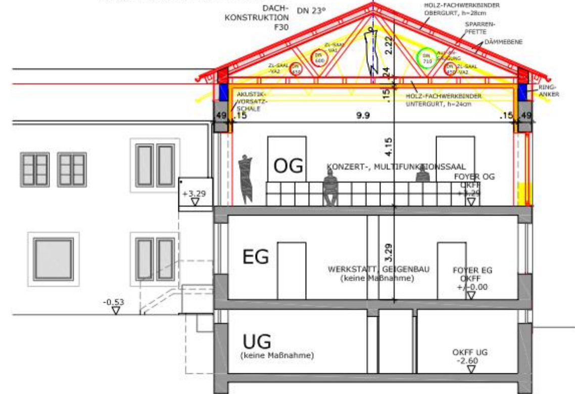
QUERSCHNITT Q-Q
